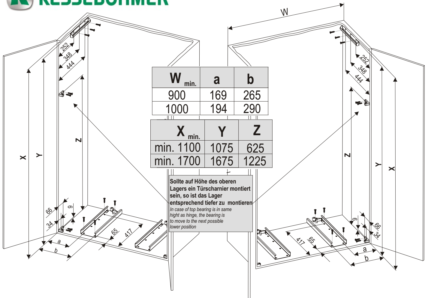
Anlieferungszustand für rechts scharnierte Tür State at delivery
